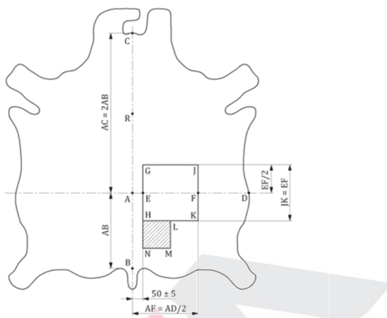
图2 家具用头层皮革取样方法
